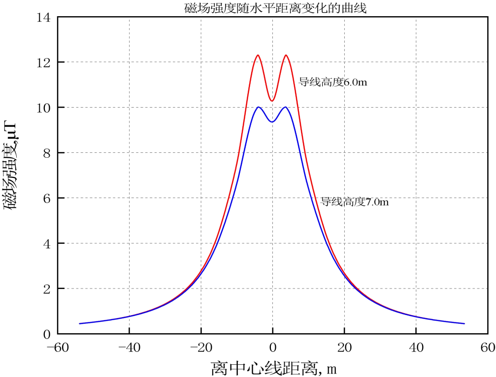
图 11 工频磁感应强度衰减趋势图
