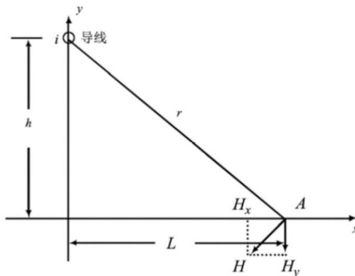
图 9 工频磁感应强度预测示意图
