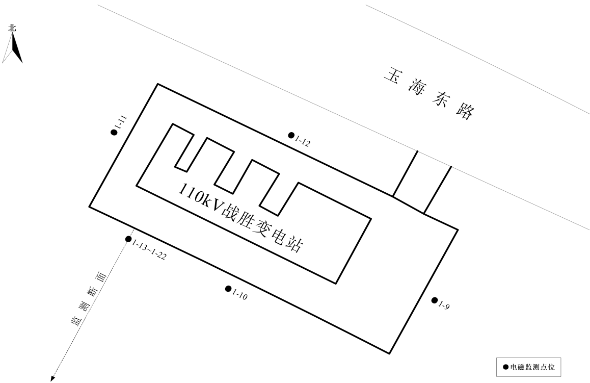
图 8 类比站厂界及衰减断面监测布点图
