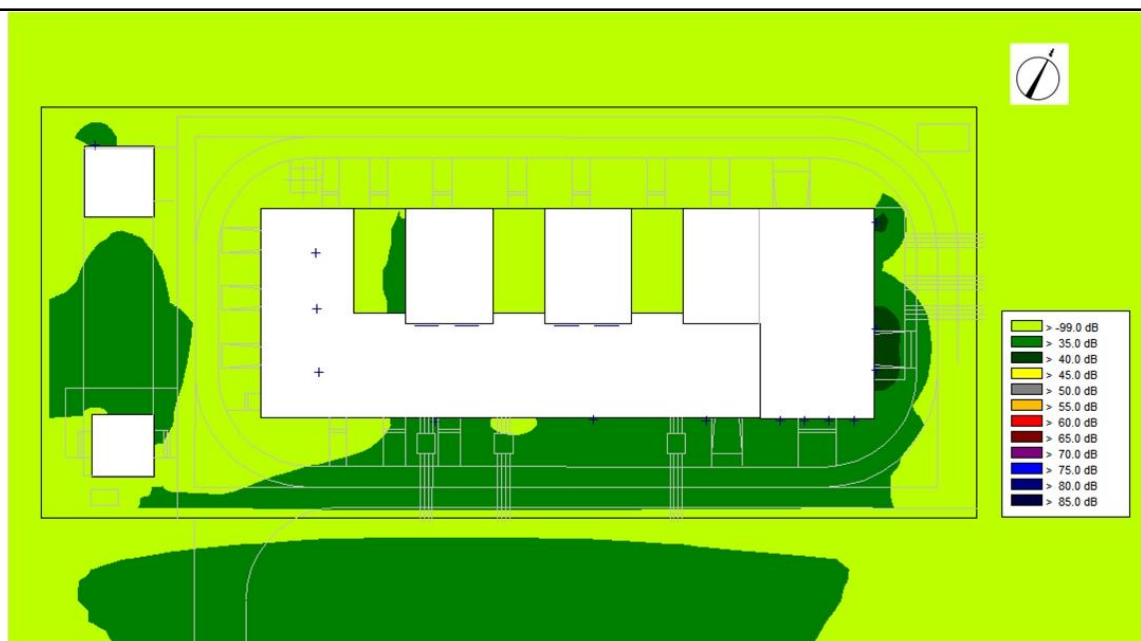
图 4-3 本项目噪声等值线分布图（离地 1.2m）
