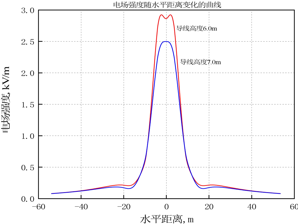
图 10 工频电场强度衰减趋势图
