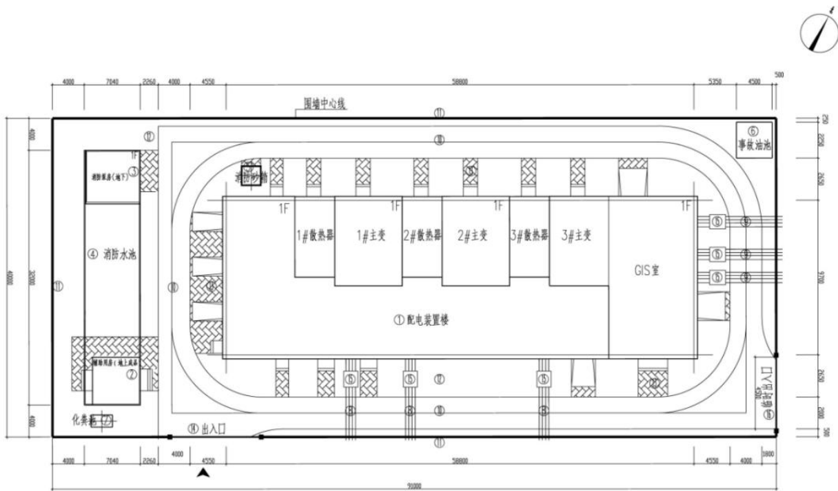
图 6 本项目拟建变电站平面布置示意图
