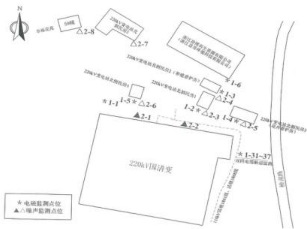
图 14 类比电缆线路监测点位示意图
