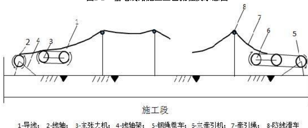
图 2-3 本项目张力牵引放线施工示意图
