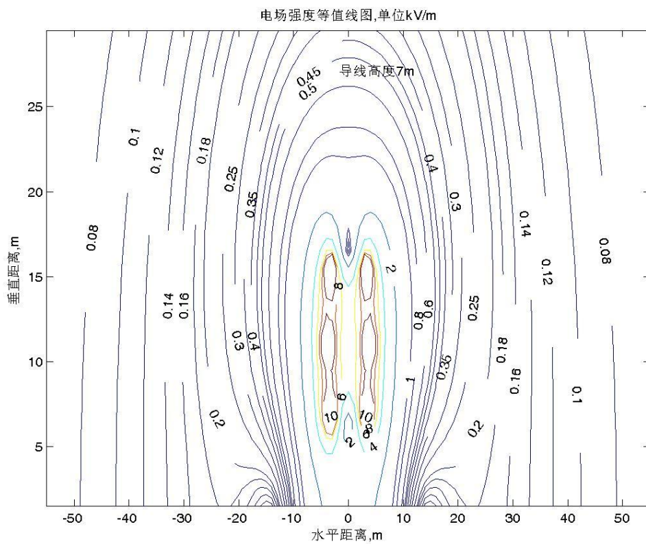
图 12 本工程 110kV 架空线路工频电场强度 4kV/m 等值线图
