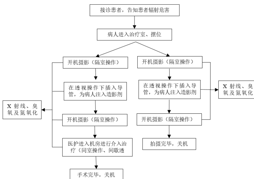
图 9-3 DSA 治疗流程及产污环节示意图
