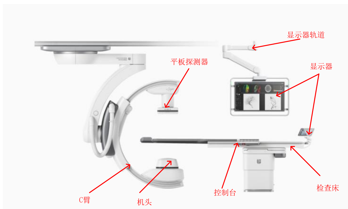
图9-1 本项目DSA外观图
