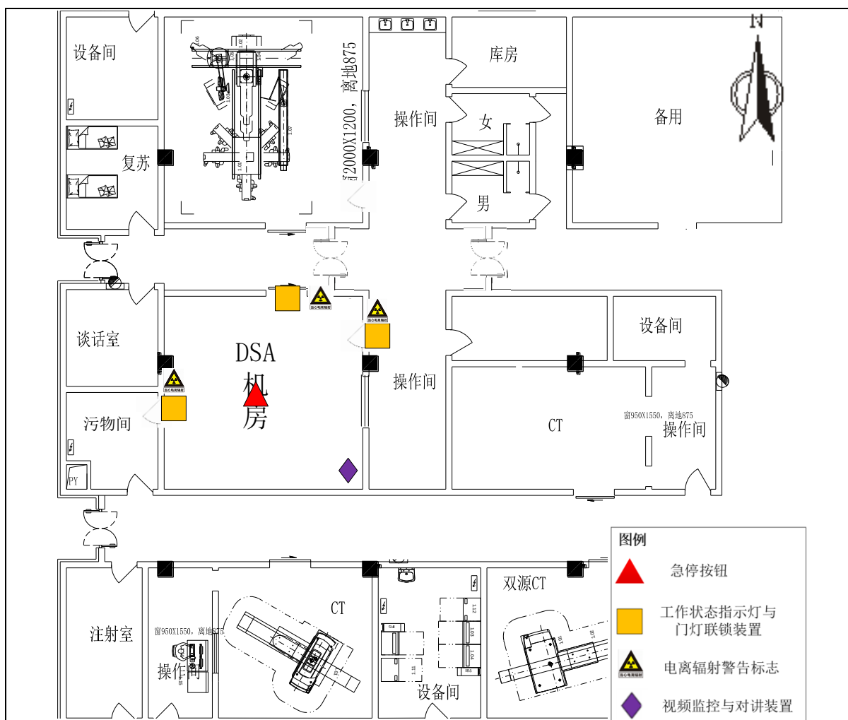
图 10-2 DSA 机房拟采取的辐射安全措施布设示意图
