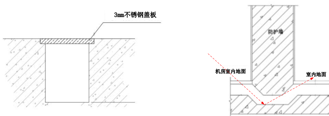
图 10-3 电缆管道示意图
